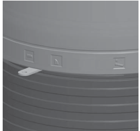
Afb. 4.11 Verbrandingsluchtschuif volledig naar links geschoven – verbrandingslucht volledig gesloten
