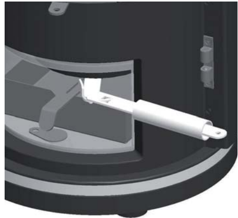
Afb. 4.16 Koolrooster bewegen om te ontassen
