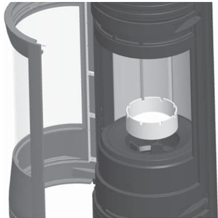
Afb. 9.1 Hittedekking in onderste houders
