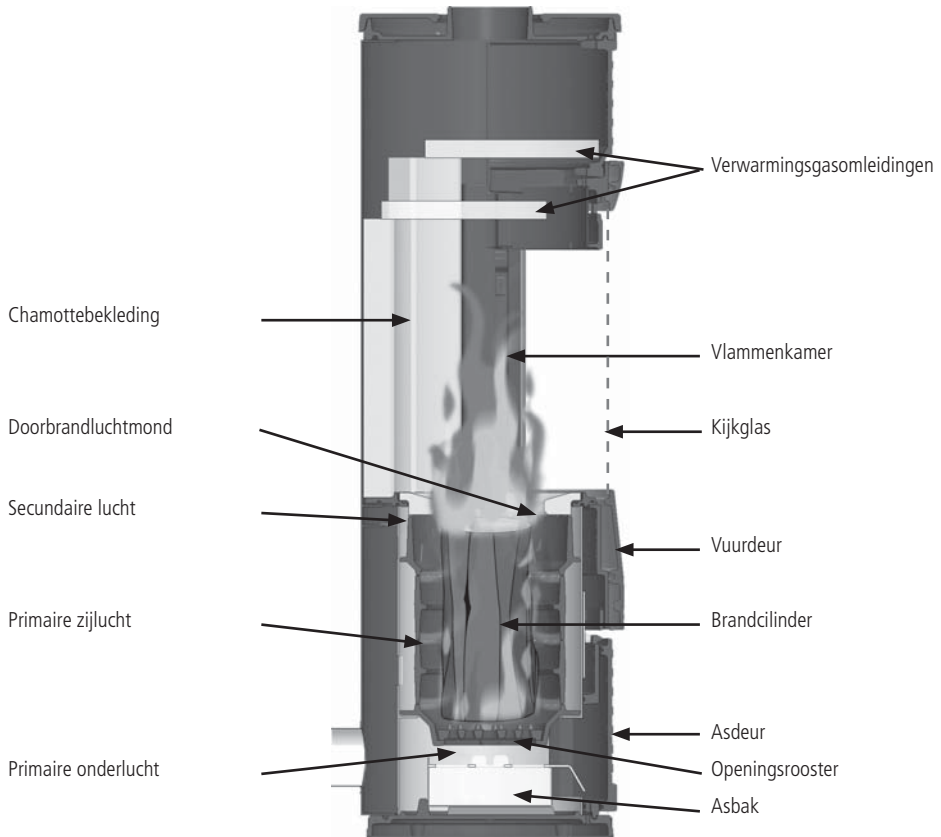
Afb. 4.1 Opbouw van de UNICA
