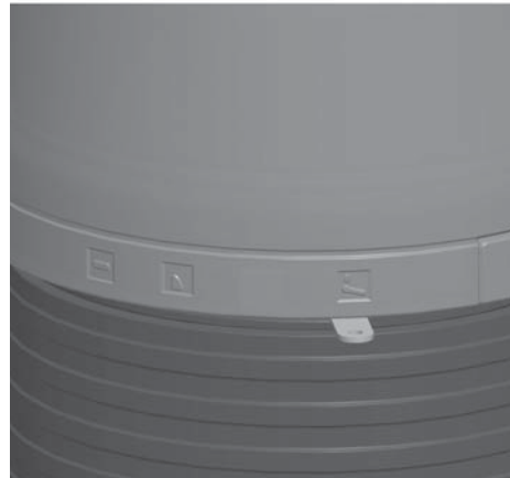
Afb. 4.10 Verbrandingsluchtschuif volledig naar rechts geschoven – verbrandingslucht volledig geopend
