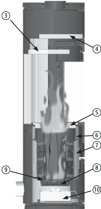
Afb. 8.2 Reserveonderdelen
