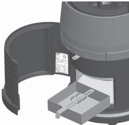
Afb. 4.3 Geopende asbakdeur
