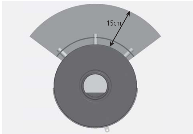
Afb. 1.2 Minimale afstanden tot brandbare bouwmaterialen of onderdelen met hitteschild
