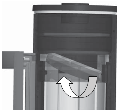
Afb. 8.3 Omleidingssteen verwijderen
