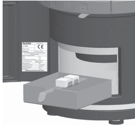
Afb. 4.9 Aanmaakhulp in de daarvoor voorziene houder op de asbak
