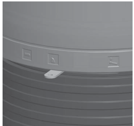
Afb. 4.12 Verbrandingsluchtschuif in het midden – normale verwarmingspositie ("nominaal verwarmingsvermogen")
