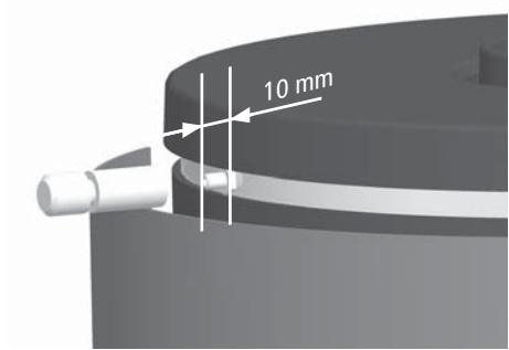
Afb. 3.5 Hittedekking in onderste houders
