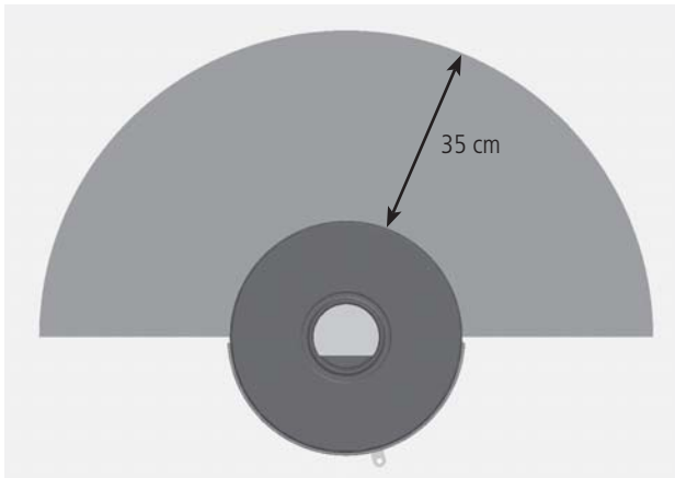
Afb. 1.1 Minimale afstanden tot brandbare bouwmaterialen of onderdelen
