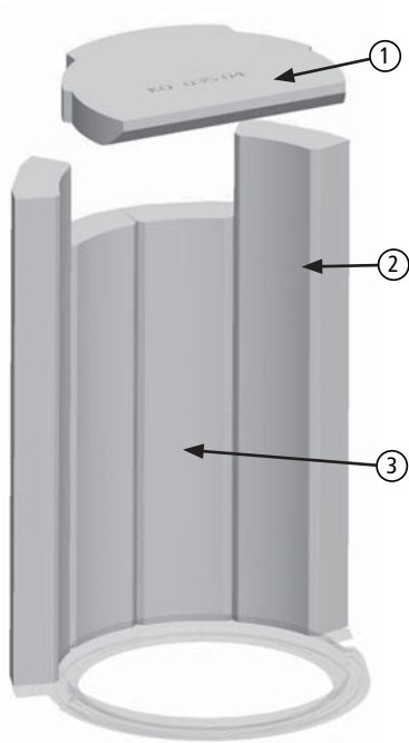
Afb. 8.1 Vuurkamerbekleding
