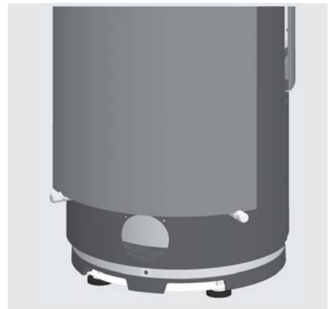
Afb. 3.4 Hitteschild in onderste houders
