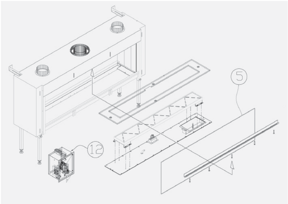
Abb. 5.2 Übersicht Bauteile
