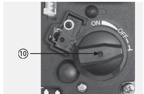
Abb. 4.21 Stellknopf des Gasreglers
