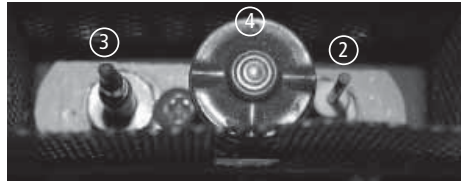
Abb. 5.1 Flammenwächter, Pilot-Brennerdüse und Zünddorn
