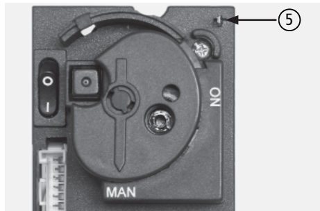
Abb. 4.18 Flachstecker-Anschluss für Piezo-Zünder am Gasregler
