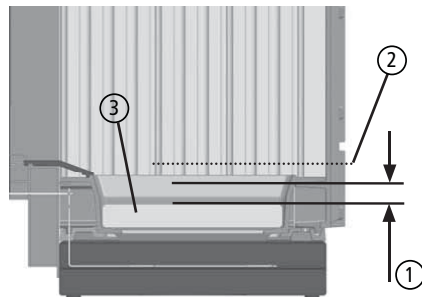
Abb. 3.14 Aschebett, Ascheniveau
